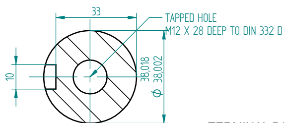
Przekrój A-A 1:1
